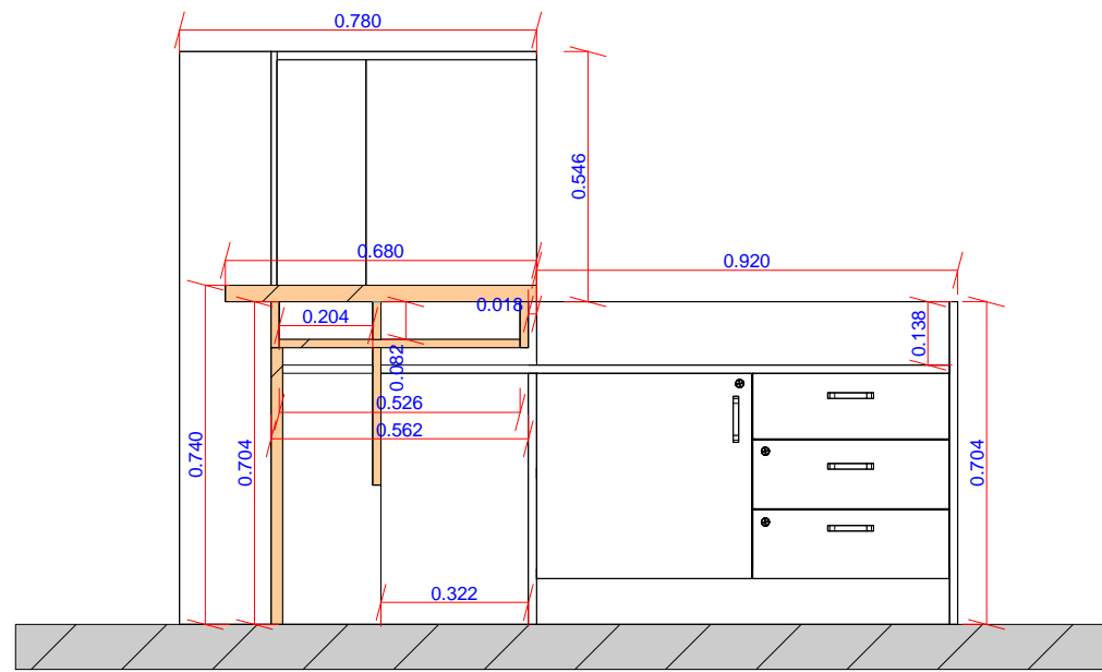
ჭრილი 2-2
