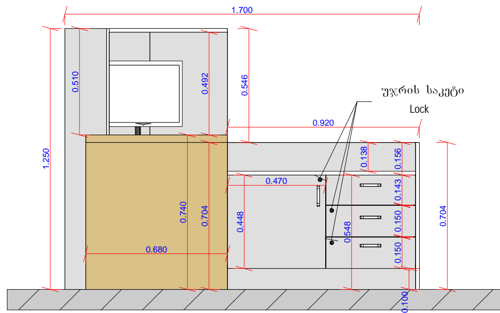
ფასადი-2
