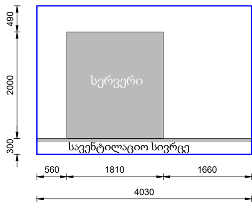
ჭრილი 3-3 მ-1:50
