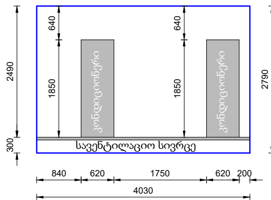
ჭრილი 3-3 მ-1:50
