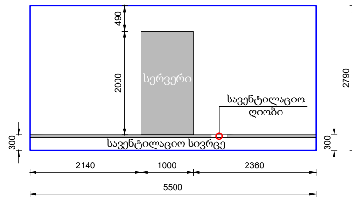
ჭრილი 4-4 მ-1:50
