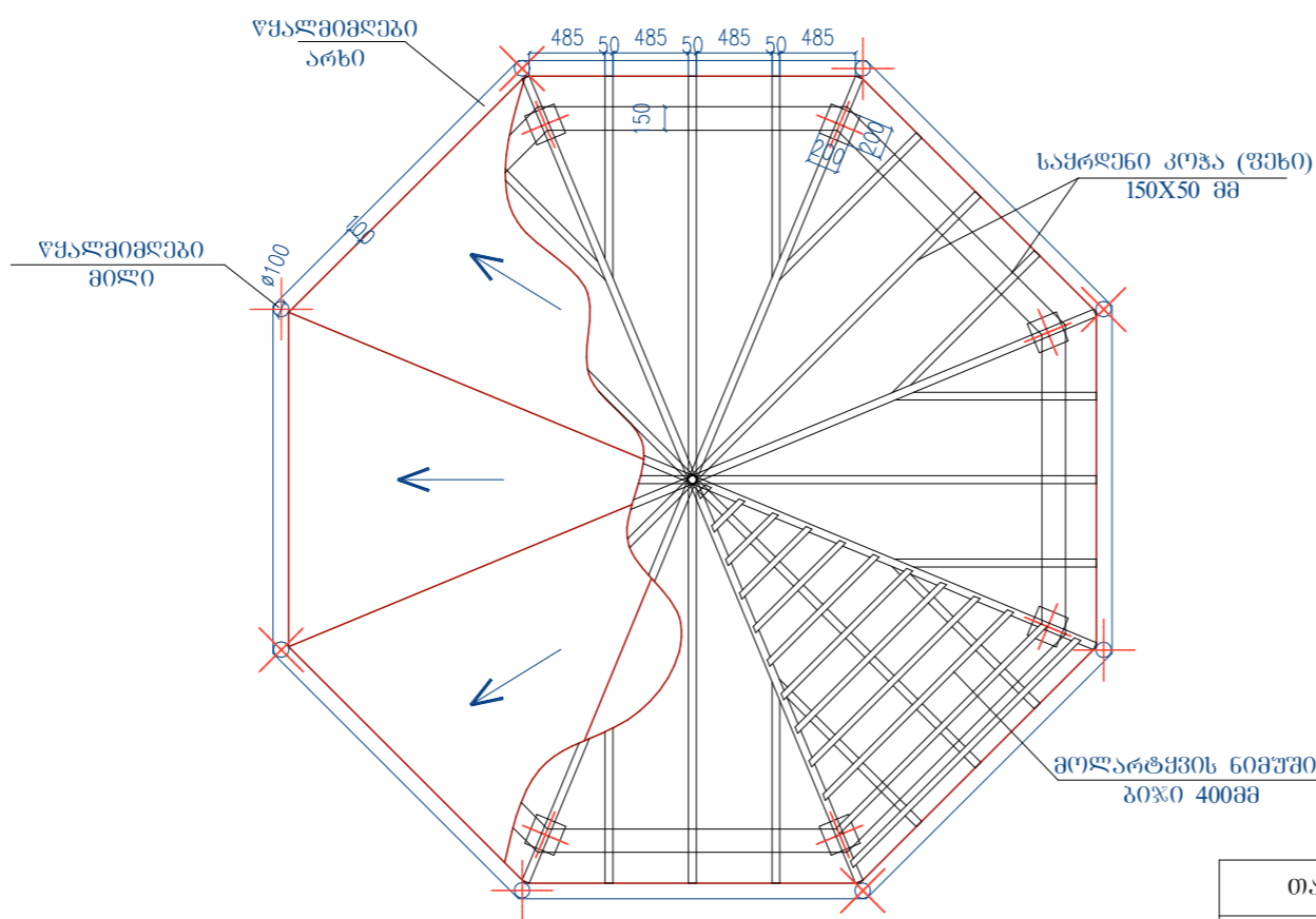
ფანჩატურის სახურავის კონსტრუქცია წყალარინება
