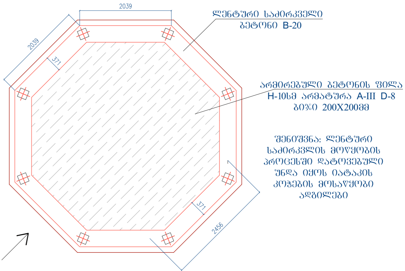
ფანჩატური ზედა ლენტური საპირკველის და იატაკის მოწყობა
