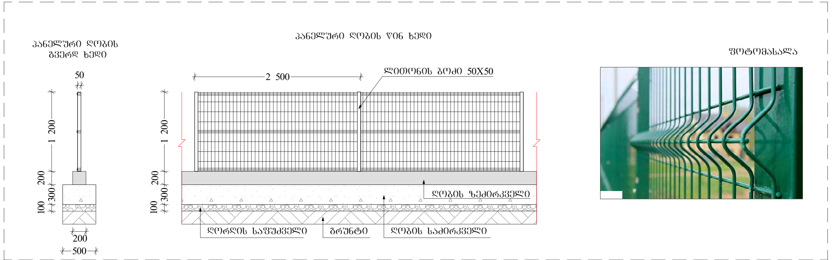
ჭიშკრის წინ სედი
