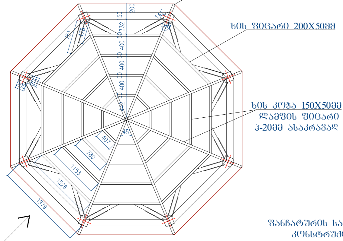
ფანჩატური ჰერის მოლარტყვა
