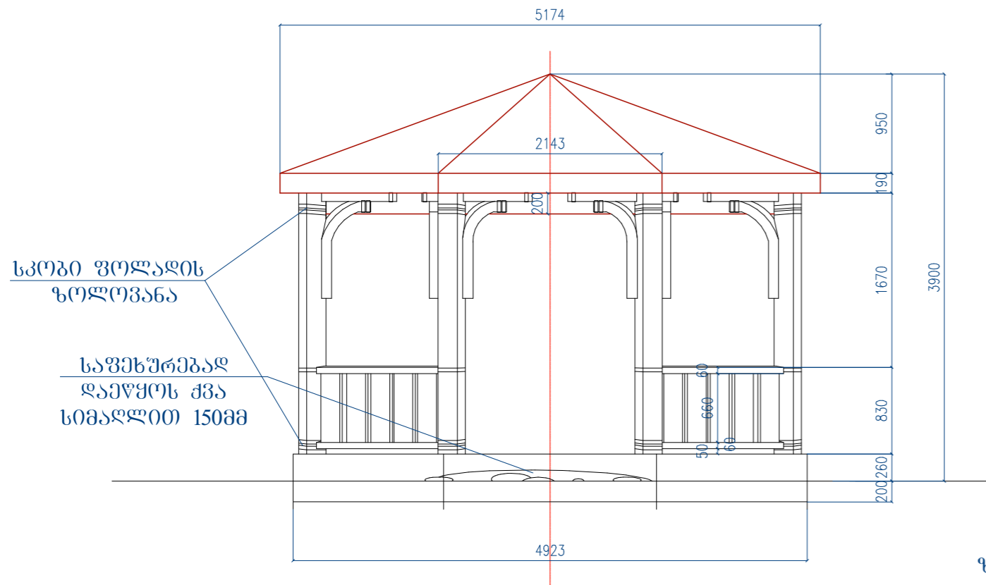
ფანჯატური ხელი შესასვლელის მხრიდან
